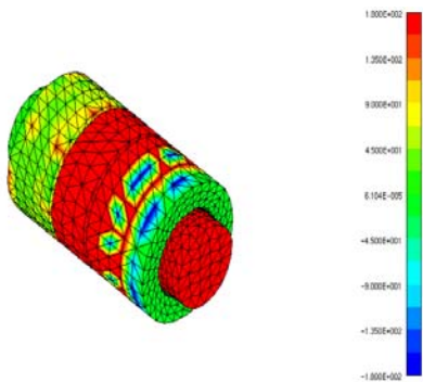
Fig. 5 1100Hz에서 음장해석
