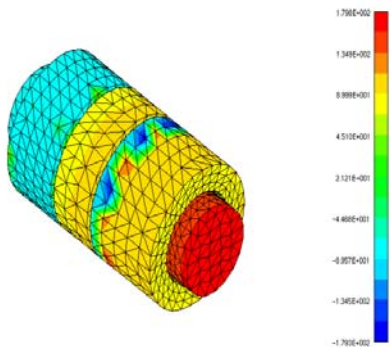
Fig. 4 700Hz에서 음장해석
