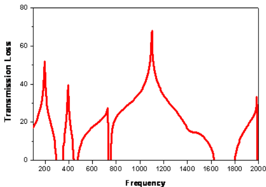
Fig. 6 시뮬레이션 해석결과
