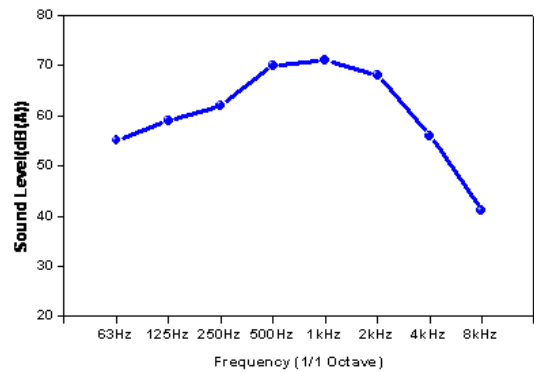
Fig. 2 팬 소음의 주파수 특성
