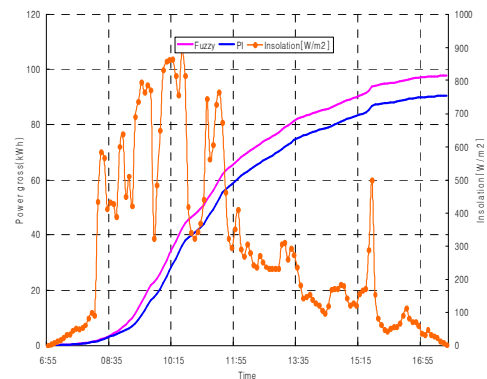
그림 8. PI제어 및 DFC에 의한 발전량(일사량 변화가 많은 환경) Fig. 8 Power gross with PI and DFC (In much changing solar radiation)
