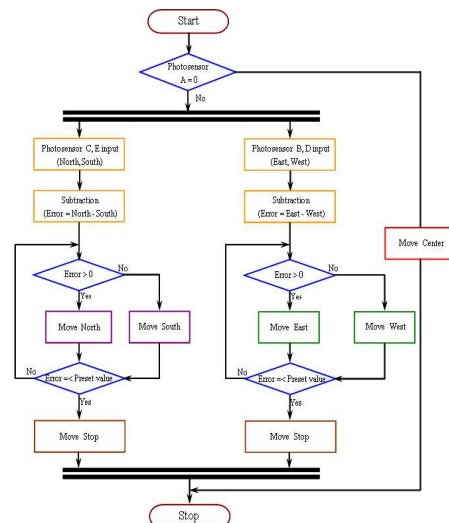
그림 4. 센서에 의한 태양광 추적 시스템의 제어 순서도.
