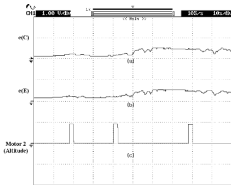
그림 6. DFC에 의한 동작특성(남-북) Fig. 6 Response characteristics of fuzzy control (south-north)
