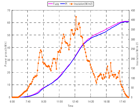
그림 7. PI제어 및 DFC에 의한 발전량(일사량 변화가 적은 환경) Fig. 7 Power gross with PI and DFC (In little changing solar radiation)
