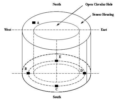
그림1. 태양위치 센서의 구조 Fig. 1 Structure of the sun position sensor
