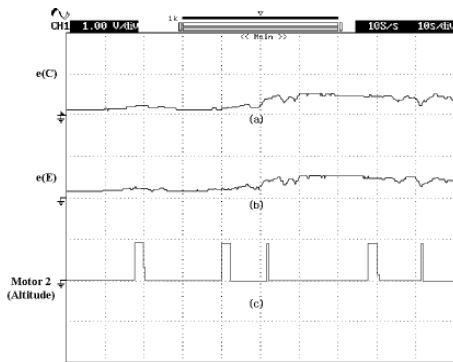
그림 5. PI제어에 의한 동작특성(남-북) Fig. 5 Response characteristics of PI control (south-north)
