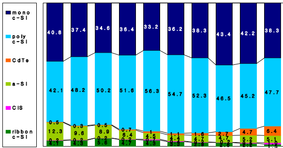
〈그림 4〉 태양전지 기술별 점유율 추이
