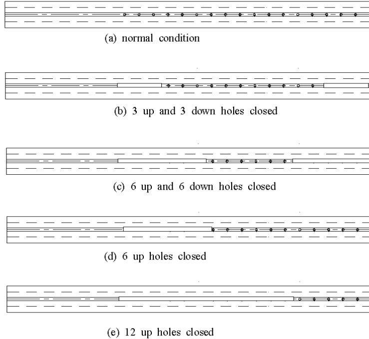
그림 4 삼각 분리 막대형 차압 유량계의 유량 특성 실험을 하기 위한 블록킹 조건
