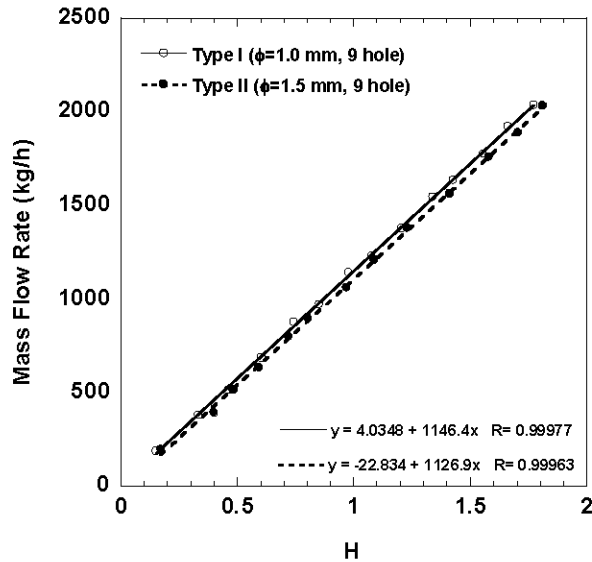
그림 3 검정 장치를 이용한 삼각 분리 막대형 차압유량계의 유량 측정 결과 (Type I and Type III)
