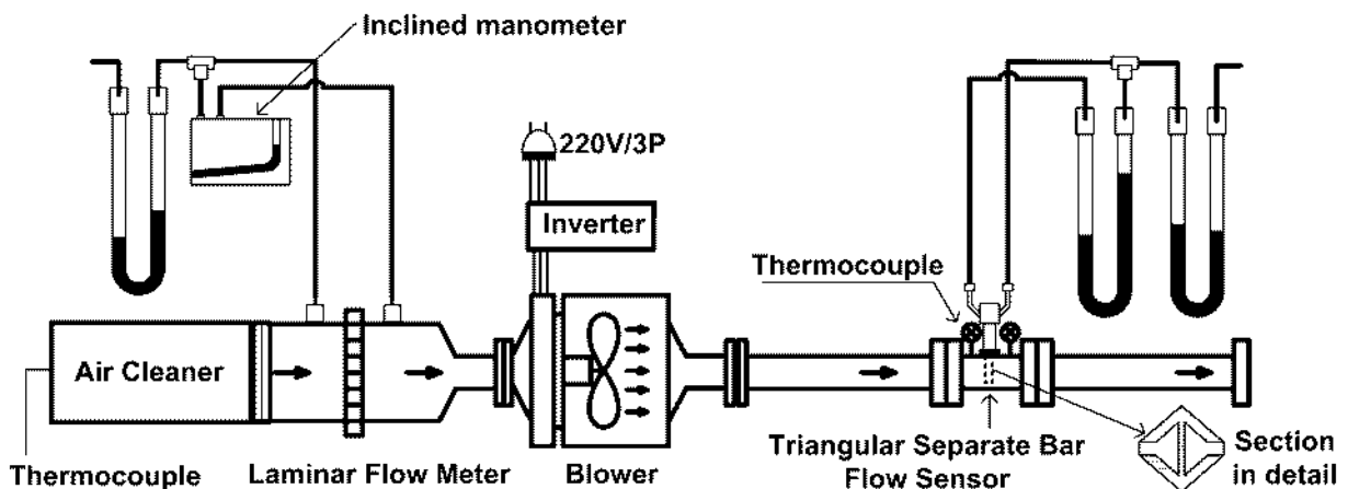
그림 1 TSB 유량계를 검정하기 위한 실험 장치 개략도
