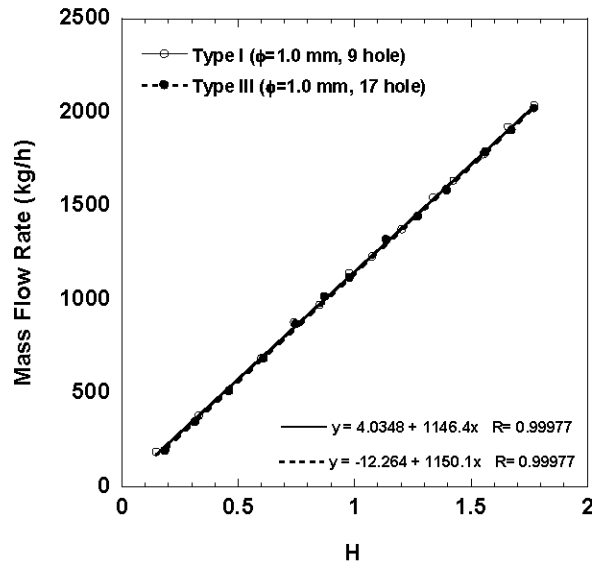
그림 2 검정 장치를 이용한 삼각 분리 막대형 차압유량계의 유량 측정 결과 (Type I and Type II)
