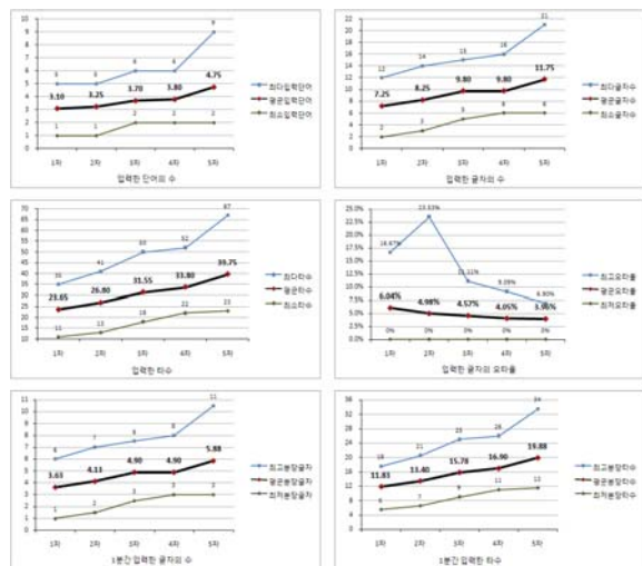
▶▶ 그림 6. 실시 회차에 따른 입력 단어, 글자, 타수, 오타율의 비교 그래프
