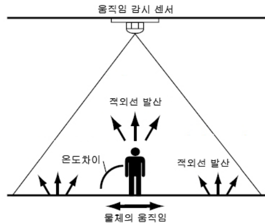
▶▶ 그림 5. 움직임 센서의 원리
