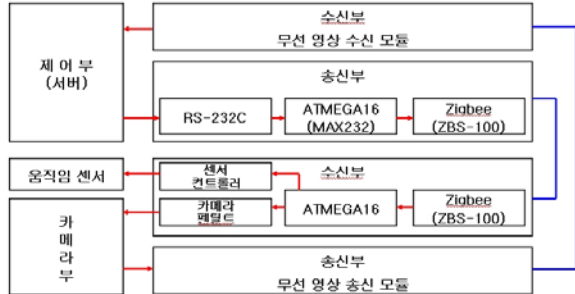
▶▶ 그림 3. 시스템 흐름도
