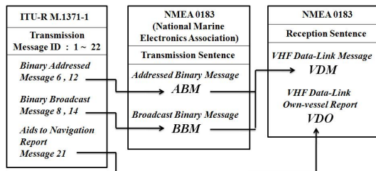
그림4 데이터전송 포맷
