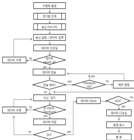
그림5 송수신 순서도
