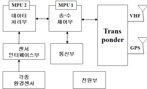
그림2 제어모듈의 하드웨어 구성도
