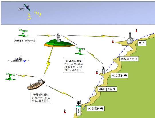
그림1 AIS와 AtoN AIS의 운용 개요 Fig.1 Application resume of AIS and AtoN AIS
