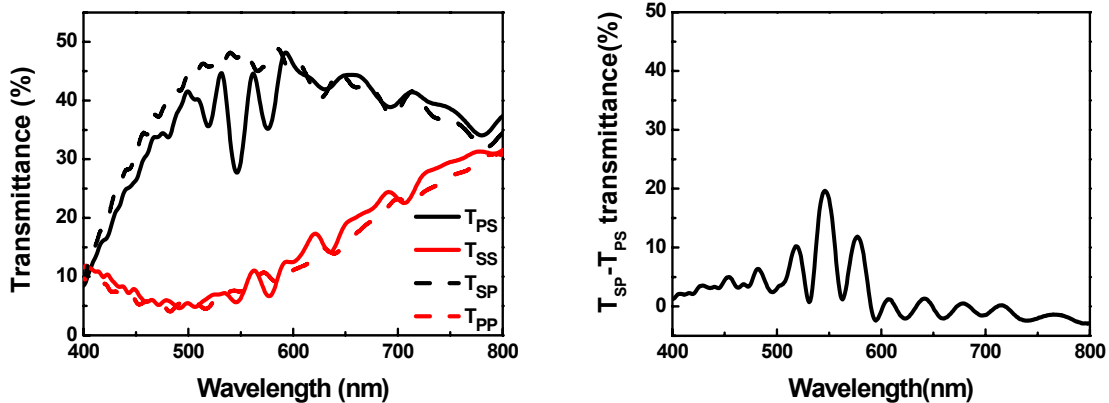
그림 2. 3층 구조의 선편광 방향변환 소자의 투과 스펙트럼: (a) T_{PS} , T_{SS} , T_{SP} , T_{PP} (b) T_{SP}-T_{PS}
