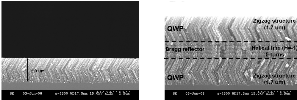
그림 1. SEM 이미지: (a) 지그재그 구조를 이용한 \lambda/4 파장판 (b) 3층 구조의 선편광 방향변환기.
