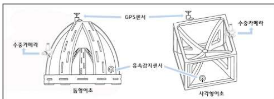
[그림 3-2] IT인공어초 설계
