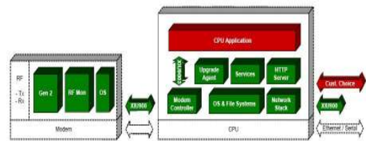
그림 1. Module construction of reader
