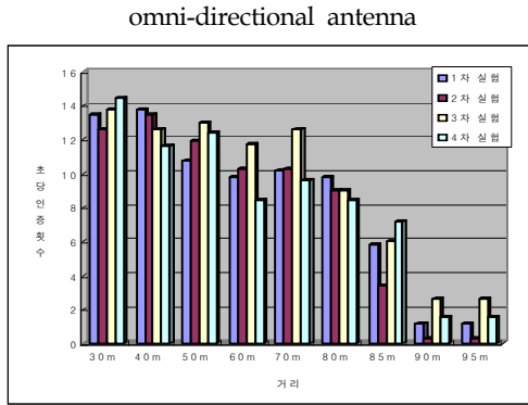
그림 7. attestation rate to distance of external directional antenna
