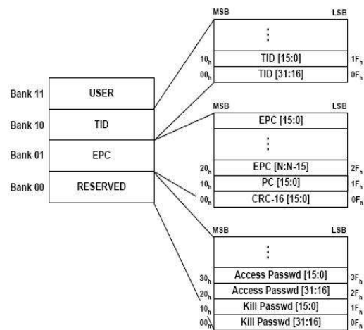
그림 2. Memory format of RF tag
