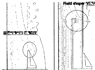
(a) Without shield (b) With field shaper 그림 2. Field shaper에 따른 전계분포.
