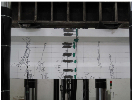
그림1. 균열 및 파괴형상
