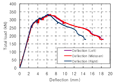
그림2. 하중-처짐 관계
