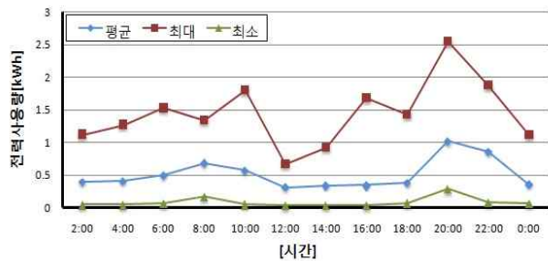
Fig. 3 J가구의 시간별 주말 전력사용량
