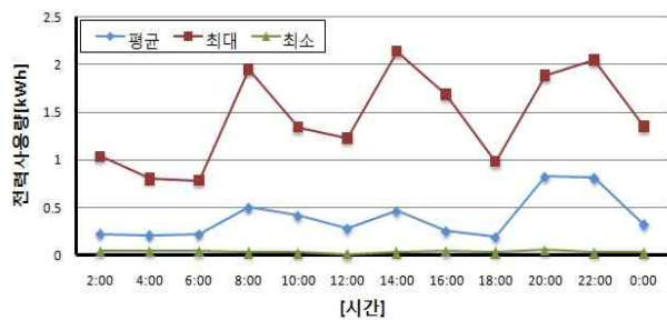
Fig. 2 J가구의 시간별 주중 전력사용량
