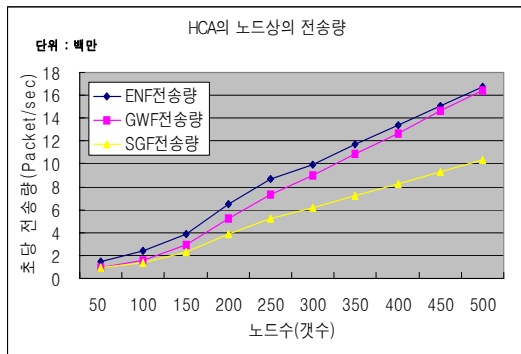
<그림3> 최고연결 알고리즘 노드상의 전송률 <Fig 3> Transmission rate of HCA
