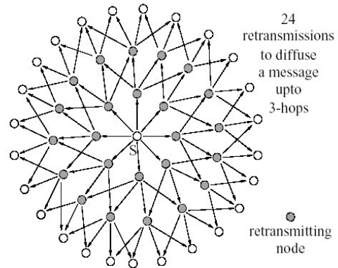
<그림 2> 클러스터링 없이 패킷 전송 <Fig2> Without clustering of packet transmission
