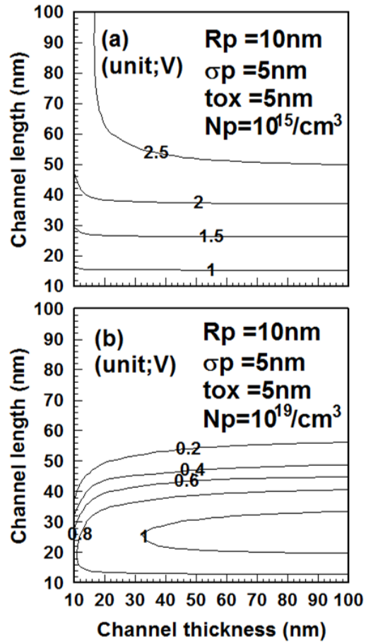
그림 3. 채널길이와 채널두께의 변화에 따른 항복전압의 변화 (a)도핑농도가 10^{15}/cm^3 일 때 (b) 도핑농도가 10^{19}/cm^3 일 때
