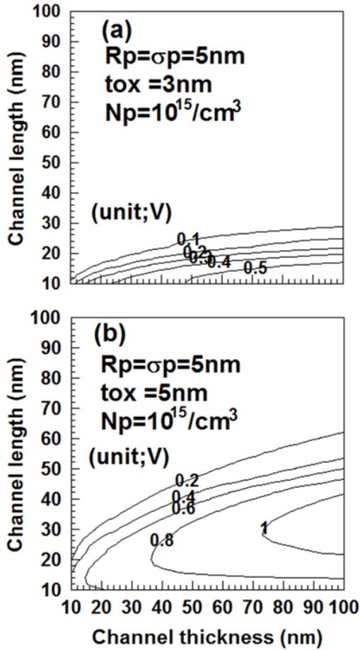
그림 2. 채널길이와 채널두께의 변화에 따른 항복전압의 변화 (a) 게이트산화막두께가 3nm일 때 (b) 게이트산화막두께가 5nm일 때
