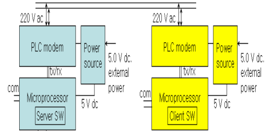
그림 7. 개발된 케이블 식별시스템 구조
