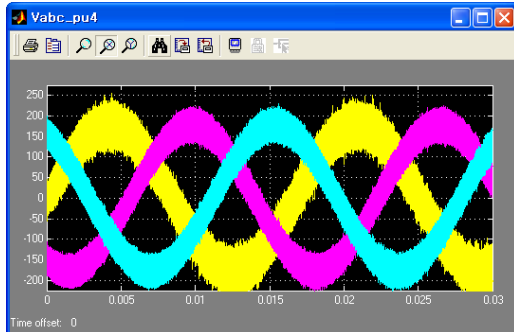
그림 5. 배전선 2차 저압측 전압신호
