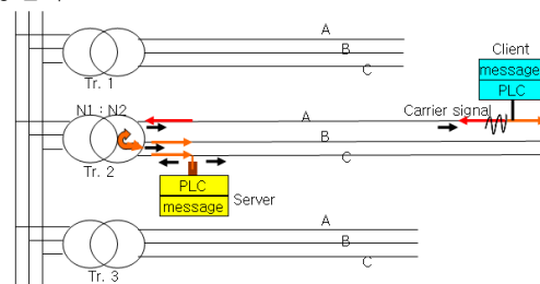
그림 2. 케이블 식별시스템 원리
