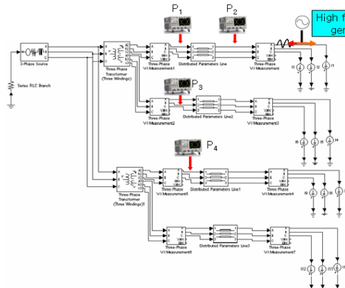
그림 4. Simulink 배전선 모델 (예)
