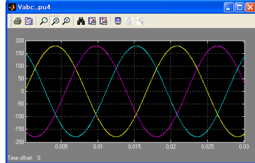
그림 6. 배전선 1차 고압측 전압신호
