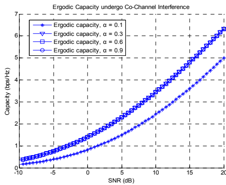
그림 2. 동일 채널 간섭 환경에서 \alpha 에 따른 채널 용량
