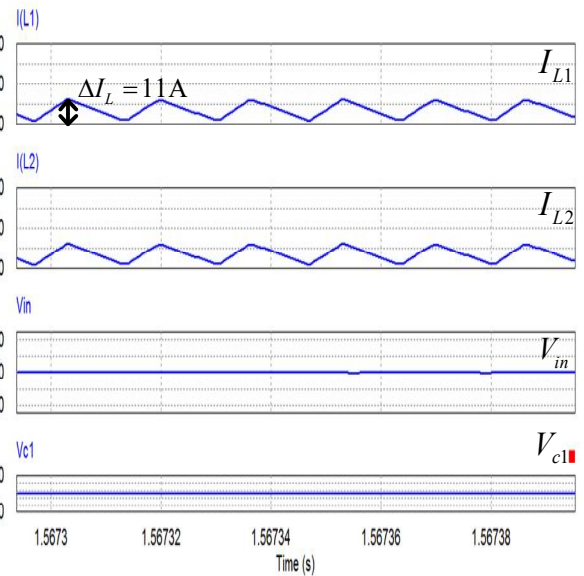
그림 4 PWM 방법을 변경한 QZSI의 시뮬레이션 결과 파형
