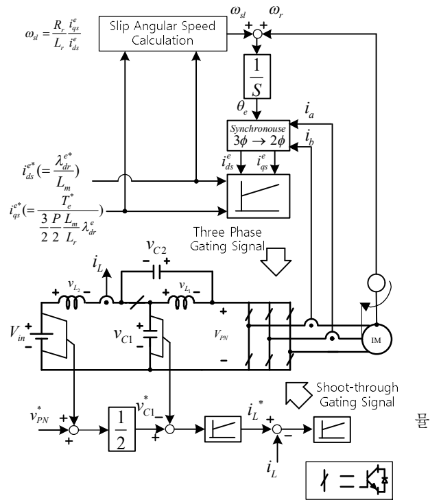
그림 1 양방향 QZSI를 이용한 모터 제어 시스템
