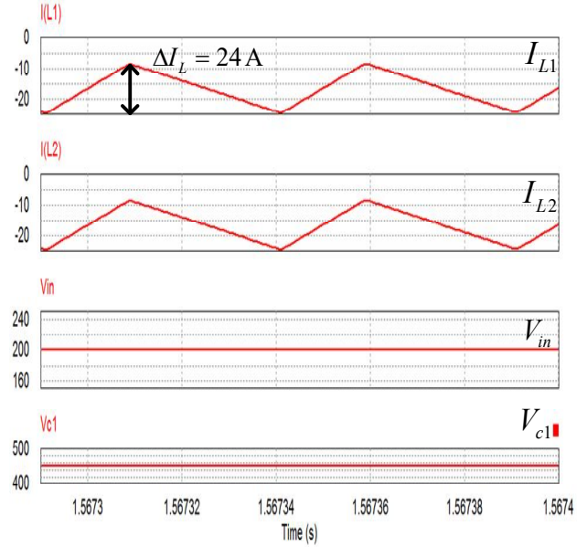
그림 3 기존의 PWM 방법을 적용한 QZSI의 시뮬레이션 결과 파형
