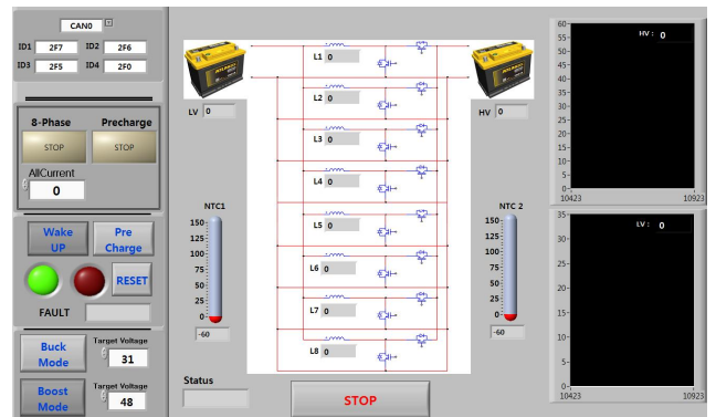
그림3. Tester Controller
