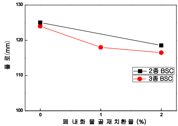
그림 1. 폐نه화물 골재에 따른 플로
