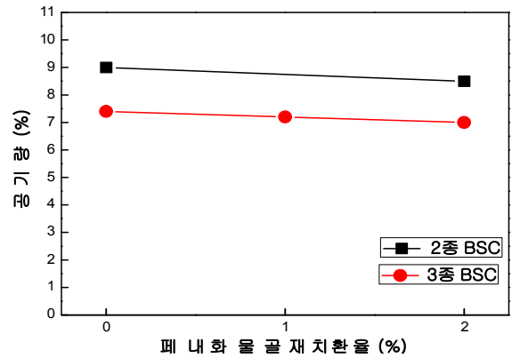
그림 2. 폐نه화물 골재에 따른 공기량
