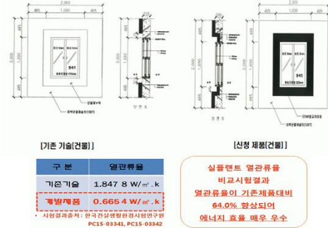
(b) 열관류율 비교 실험
