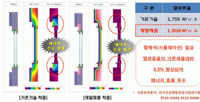
(a) 열관류율(전열해석 프로그램)
