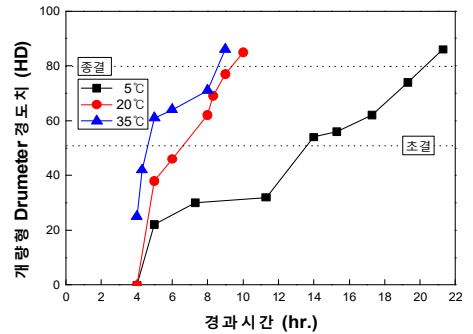
그림 3. 시간경과에 따른 개량형 Durometer의 경도치
