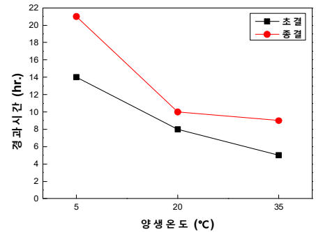
그림 2. 양생온도 변화에 따른 초결과 종결시간
