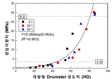
그림 4. 관입저항치와 개량형 Durometer의 상관관계
