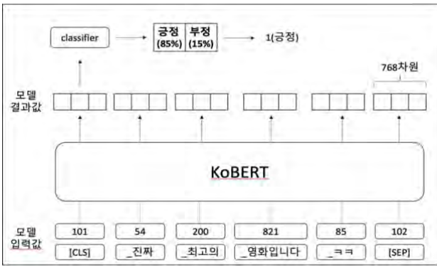
(그림 1) KoBERT 모델을 이용한 감정 분석 시스템
