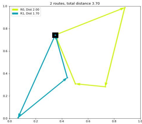
(a) VRP(n=5)
