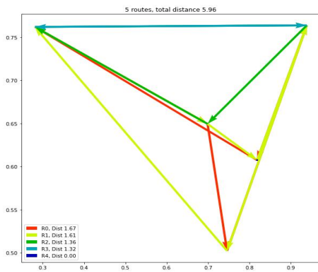
(b) GVRP(n=5)
