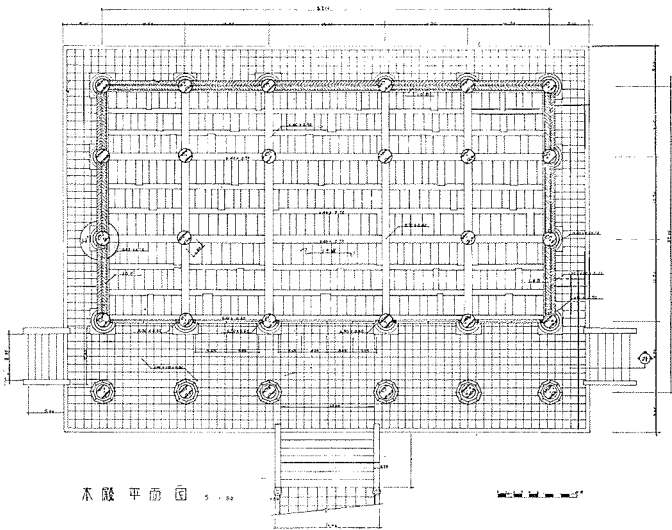
本殿 平面圖
