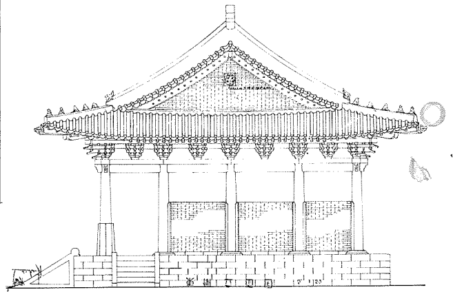
東側 立面圖
