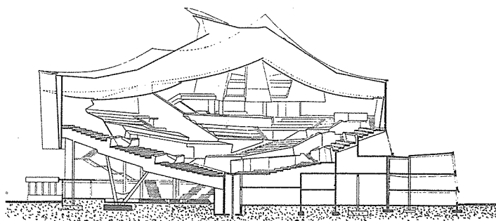
베를린 필하모니홀 (콘크리트) 断面
