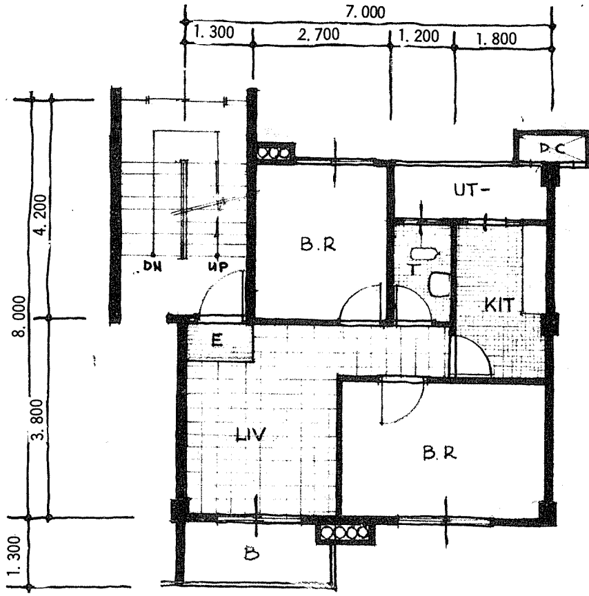
15평형 평면도 SCALE 1 : 100 잠 실 아파트
