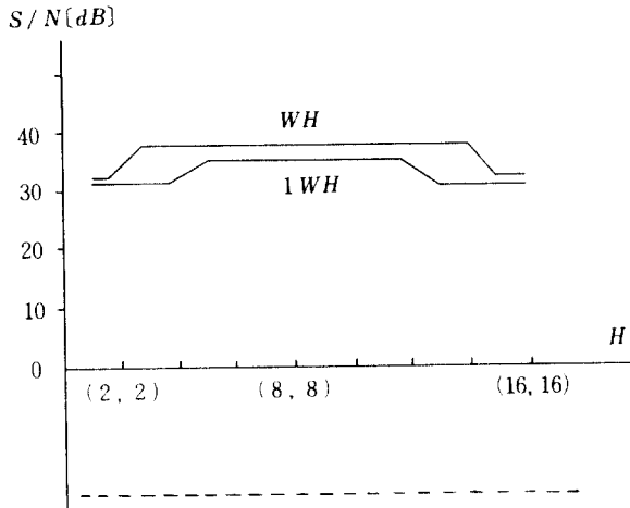
그림 5 16×16블록에서 WH와 LWH의 신호대 잡음비 SNR comparison between Hadamard and LWH in 16×16 block.
