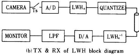
그림10 LWH의 연산알고리즘과 전송도 LWH transform circuit and its calculation algorithm.
