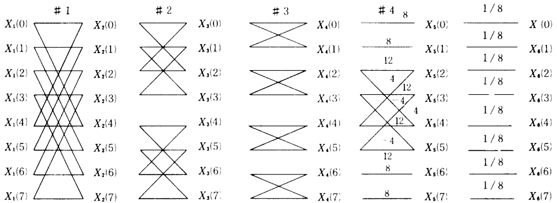
그림 2 고속 LWH 신호흐름선도, N=8 Fast LWH signal flow graph, N=8 .
