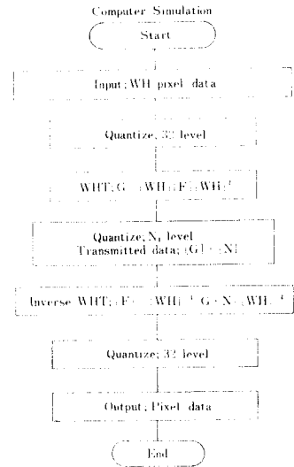
그림 6 영상처리 순서도 Flow chart of image processing
