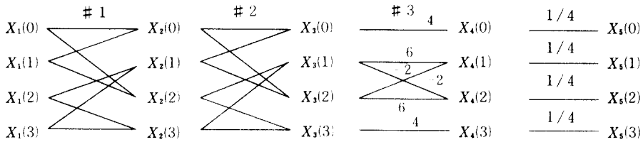
그림 1 고속 LWH 신호흐름선도, N=4 Fast LWH signal flow graph, N=4
