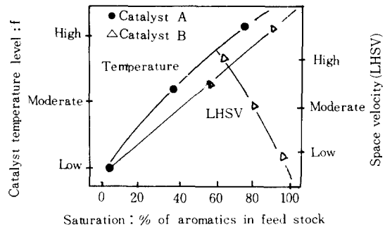
그림 3. 飽和反應에 미치는 촉매, 액공간속도 및 촉매온도의 영향
