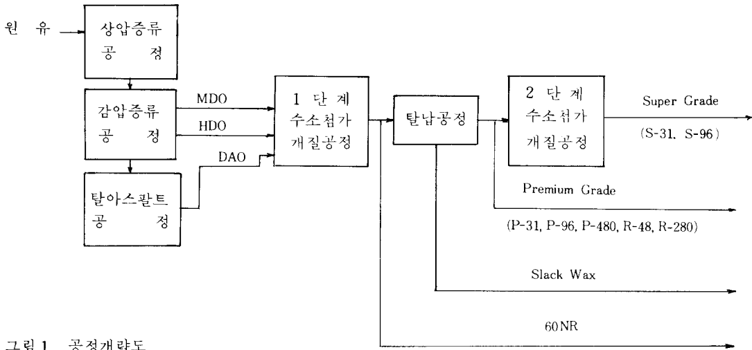
그림 1. 공정개략도
