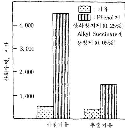
그림 6. 산화방지제 첨가효과비교
