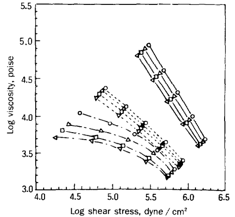
Fig. 9. Effect of shear intensity on viscosity for EPDM/PP blend at 200°C (DCP concn ; 0.67 phr) : (—) 25 : 75 PP : EPDM ; (···) 50 : 50 PP : EPDM ; (-·-·) 75 : 25 PP : EPDM (○) 20 rpm ; (△) 40rpm ; (□) 60 rpm ; (▽) 80 rpm
