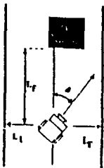
그림 2-2 퍼지 입력변수
