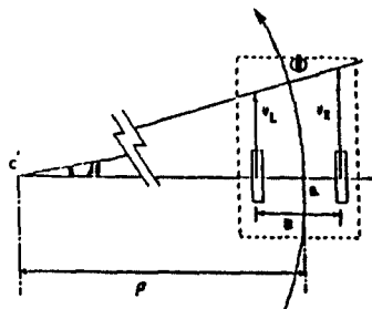
그림 4-1 2자유도(2DWIC) 이동로봇트
