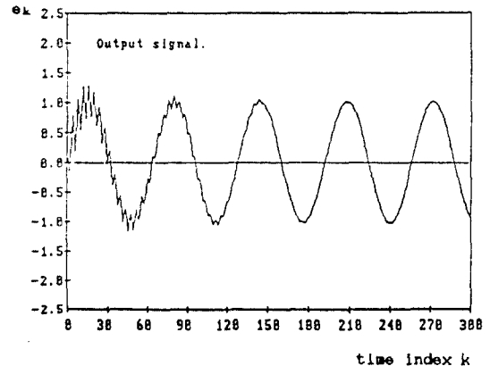
그림 7. 그림 2 ANC 모형에서의 출력 신호파형. ( k_0=0 , k_1=0 , k_2=0 ). Fig. 7. The output signal wave form of ANC model in fig.2. ( k_0=0 , k_1=0 , k_2=0 )
