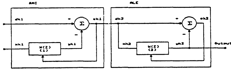
그림 3. 적응잡음제거기와 적응신호증가기 결합모형 Fig. 3. The combined model of ANC-ALE.
