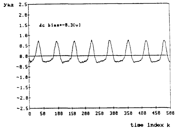
그림 16. 그림 3의 모형에서 ANC ALE 출력신호. (dc bias=-0.3[v]) Fig. 16. The output signal of ANC ALE in the model of fig.3.(dc bias=-0.3[v])
