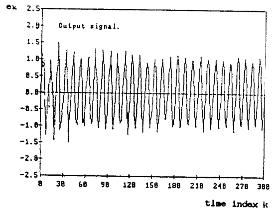
그림 12. 그림 11.의 입력신호에 대한 ANC 출력신호. Fig. 12. The ANC output signal for the input signal of fig.11.
