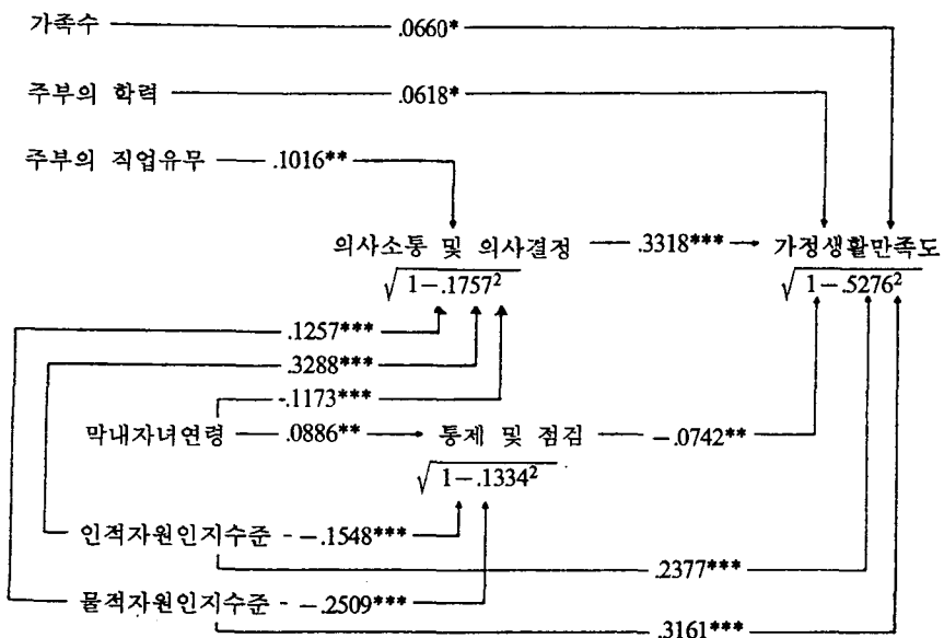
그림 2. 인과모형.
