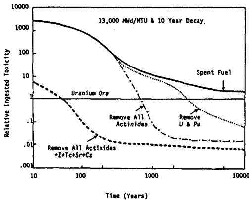
그림 2. 사용후 핵연료와 소멸처리후 방사성 폐기물의 시간에 따른 독성 비교
