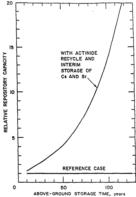
그림 3. 스트론튬 및 세슘의 균분리후의 지상보관 시간 변화에 따른 지중매몰 처분용량 변화
