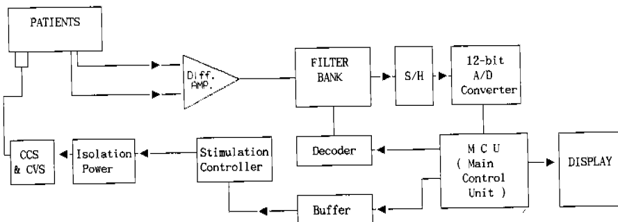
그림 1 전체 시스템의 블럭선도
