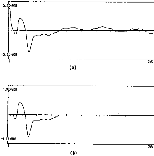
그림 7 정전압원 신경자극기에서의 파형 (a) 자극 artifact 에 오염된 신호 (b) 자극 artifact 가 제거된 신호
