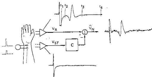
그림 5 정전류원 신경자극기에서의 자극 artifact 제거를 위한 블럭선도
