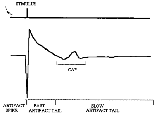
그림 3 복합활동전위 신호
