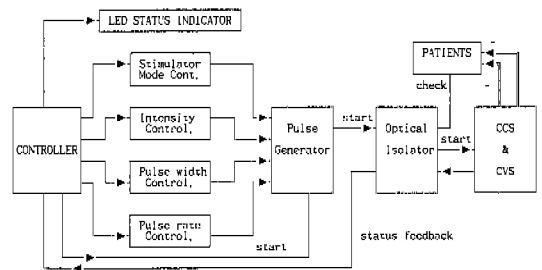
그림 2 신경자극기의 블럭선도
