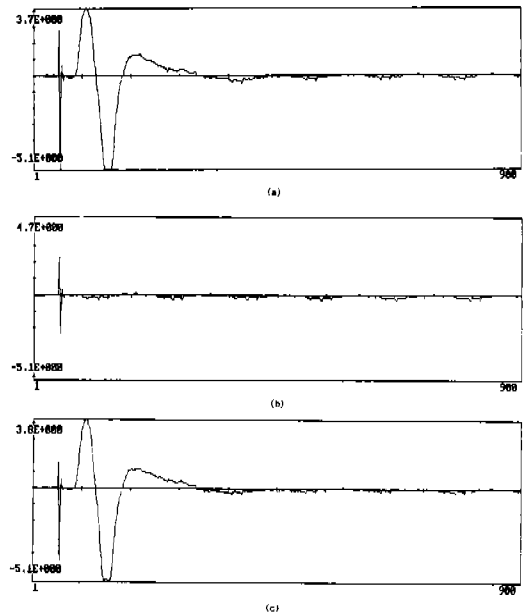
그림 8 정전류원 신경자극기에서의 파형
