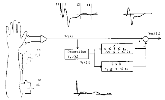
그림 4 정전압원 신경자극기에서의 자극 artifact 제거를 위한 블록선도
