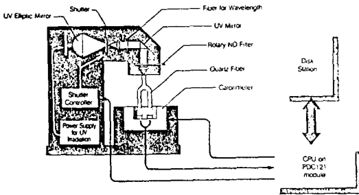
그림 16. PDC의 구조.
