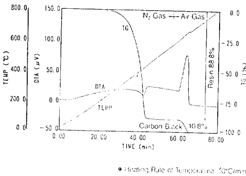
그림 4. Toner중의 carbon black함량 측정 TG/DTA thermogram.
