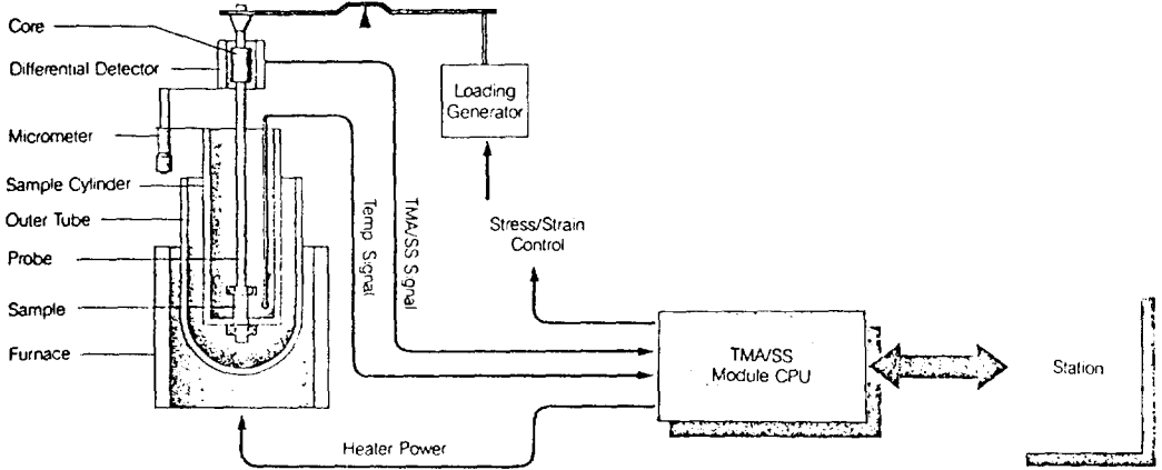
그림 15. TMA/SS 구조도.
