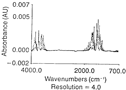
그림 7. 60°C에서 발생한 가스의 IR spectrum.
