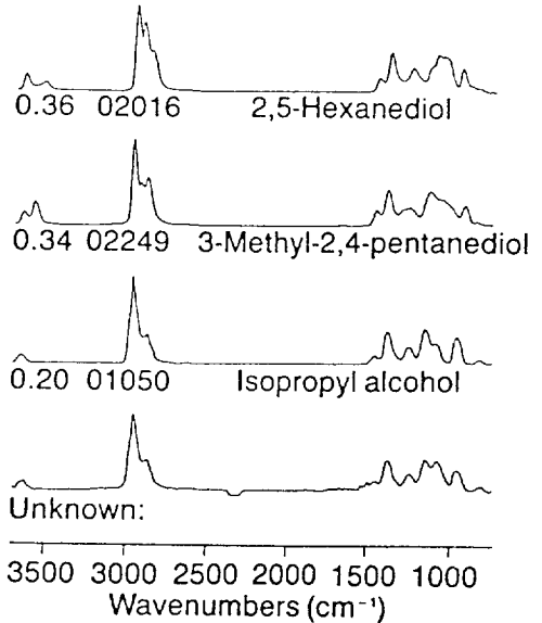
그림 8. 135°C에서 발생한 가스의 IR spectrum과 library search 결과.
