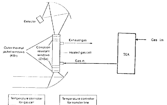
그림 5. TGA/FT-IR 구조도.
