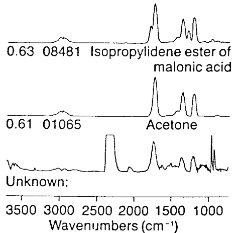
그림 9. 175°C에서 발생한 가스의 IR spectrum 및 library search 결과.
