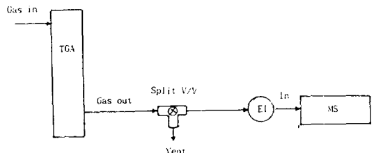
그림 14. TGA/MS 구조도.
