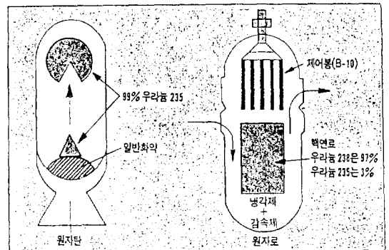
원자로와 원자폭탄 비교
