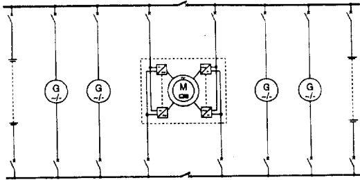
1990년대 이후 전기추진 시스템
