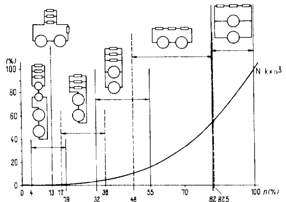
추진전지와 추진모터의 조합에 따른 속도단계
