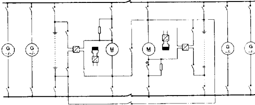
1980년대 전기추진시스템
