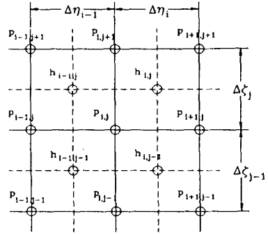
Fig. 5. Mesh for analysis ( 1 \leq i \leq \text{NET} , 1 \leq j \leq \text{NZT} )
