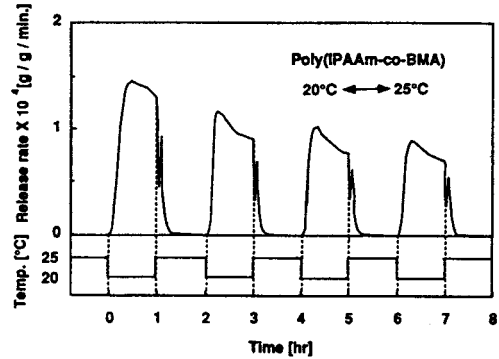
그림 4. On-off release profile of indomethacin from poly(NiPAAm-co-BMA) gel.
