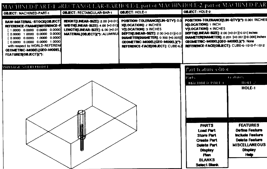
그림 9 객체 지향형 프로그램 환경이 제공하는 대화식 그래픽 도구를 이용하여 구축한 시스템 레이아웃의 한 예
