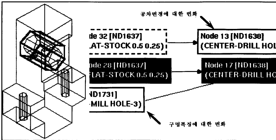
그림 5 기본적인 설계에서 두 개의 특징 형상(HOLE)을 변경하였을 때 이전 정보를 재사용한 후의 시스템 결과, 가공 허용 오차의 증대로 센터 드릴공정이 추가되었고 지름의 변경으로 마땅한 드릴 공구가 없어 밀링으로 대체되었다.
