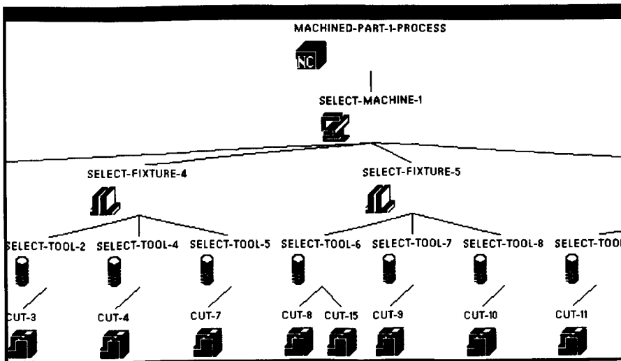
그림 3 지식베이스시스템의 중앙에 저장된 공정정보의 연관관계 및 가공순서 정보
