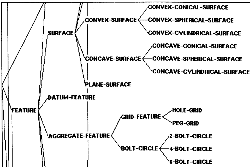
그림 7 절삭가공용 지식베이스엔지니어링 시스템[NextCut, 이수홍 1991]내에 정의된 부품 객체들의 일반적 계층 구조도
