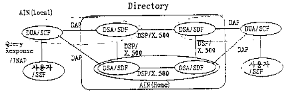
(그림 6) X.500과 AIN 기능간의 관계(AIN 연동) (Fig. 6) Relationship between X.500 and AIN functional model(AIN internetworking)
