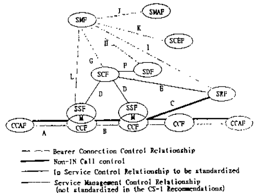
(그림 1) 지능망 기능 모델 (Fig. 1) Functional model of Intelligent Network(IN)
