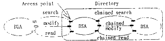
(그림 4) 분산 디렉토리 모델의 객체 (Fig. 4) Objects of the distributed Directory model
