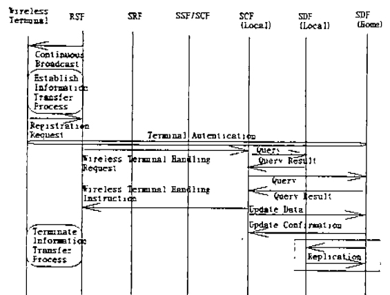
(그림 8) 위치 관리 서비스의 정보 흐름(X.500 위임 동작) (Fig. 8) Information flows of location management service(Referral operation of X.500)
