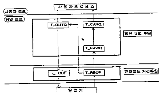
(그림 1) 단말기 인터페이스에서 사용하는 버퍼들 (Fig. 1) Buffers for TTY interface
