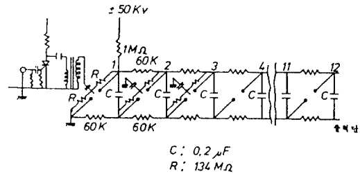
그림 3. Marx Generator 배선도. C: 0.2 \mu\text{F} R: 134 \text{ M}\Omega
