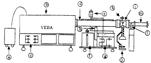
Ⓐ: 전원장치 Ⓑ: Marx 뱅크 Ⓒ: 절연유 순환기 Ⓓ: 펄스 형성라인 Ⓔ: 수면계 Ⓕ: 물탱크 Ⓖ: 물 순환기 Ⓗ: 이온 교환수지 Ⓛ: 이극관 Ⓜ: 진공펌프 Ⓟ: 게스 주입 밸브 Ⓡ: 자석 Ⓢ: 이온 전파관
