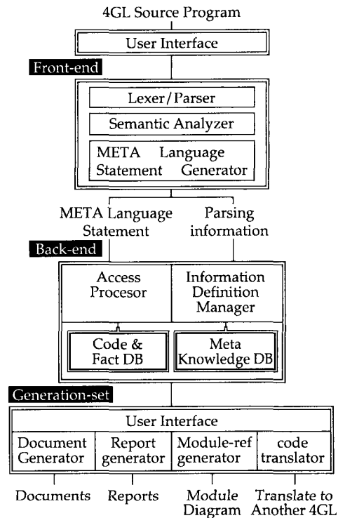
(그림 2) 전반적인 시스템 구조
