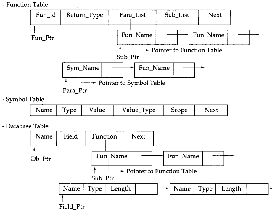
(그림 3) 파싱 정보의 자료 구조
