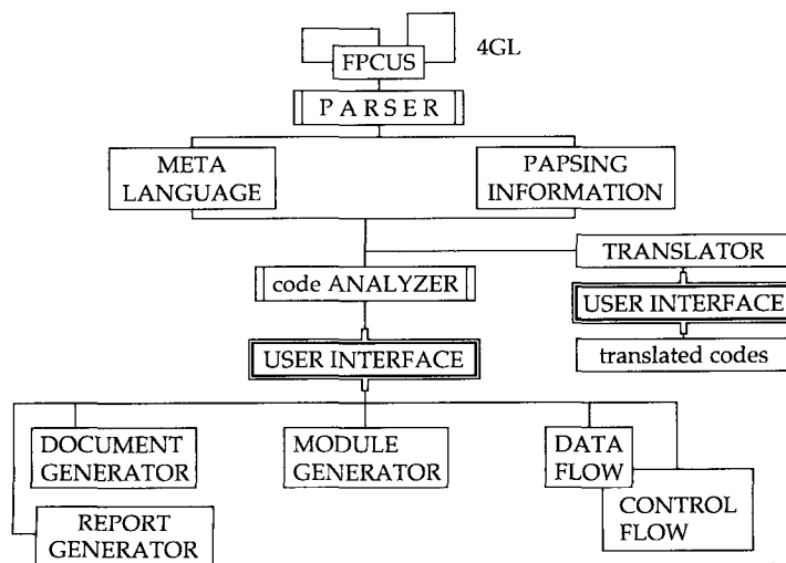
(그림 1) 전체 시스템의 구성
