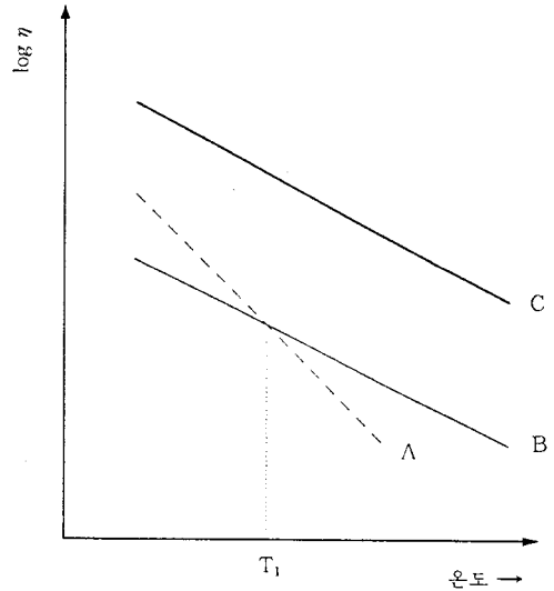
그림 2. HM형 접착제의 온도별 용융점도 변화 비교.
