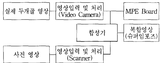
그림 16. 실험 장치 구성
