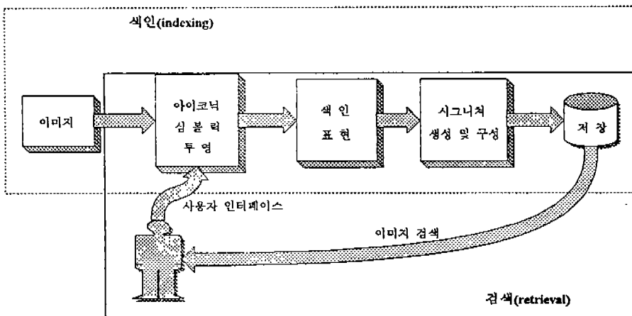
(그림 8) 공간 매치 검색 시스템 구성도 (Fig. 8) The diagram of spatial match retrieval system
