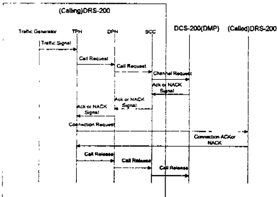
(그림 9) 시뮬레이션의 호처리 과정 (Fig. 9) Call Processing Procedure of Simulation
