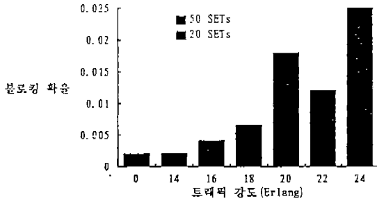
(그림 11) 입력 트래픽에 따른 블로킹 확률 (Fig. 11) Blocking probability relative to input traffic
