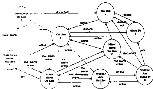
(그림 4) 다음 상태를 결정하는 상태천이도 (Fig. 4) State Transition Diagram for Next State
