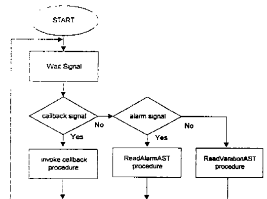
(그림 8) 그래픽 서버 알고리즘의 순서도 (Fig. 8) Flow chart of graphic server algorithm
