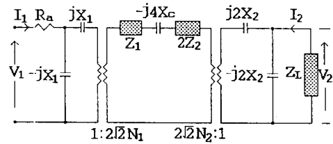
그림 5. 기본 공진주파수 부근에서 복합 압전 트랜스듀서의 등가회로
