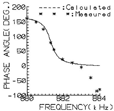
그림 12. 주파수와 위상차의 관계 Fig. 12. Phase angle to the frequency.
