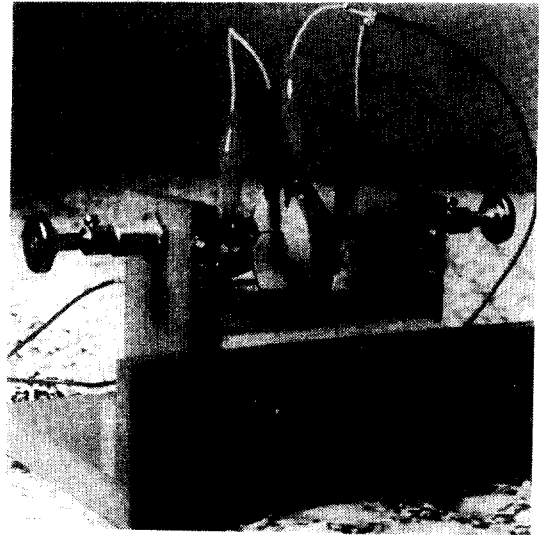
그림 6. 지지장치를 포함한 복합 압전 트랜스듀서 Fig. 6. A composite piezoelectric transducer with a supporting device.
