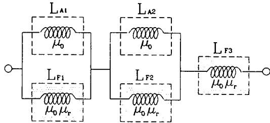
[그림 4] 합성인덕턴스 모델 [Fig. 4] A synthesized inductance model.
