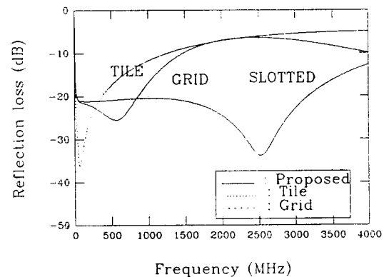
〔그림 7〕 Case 2(표 1)의 전파흡수체에 대한 반사주파수 특성
